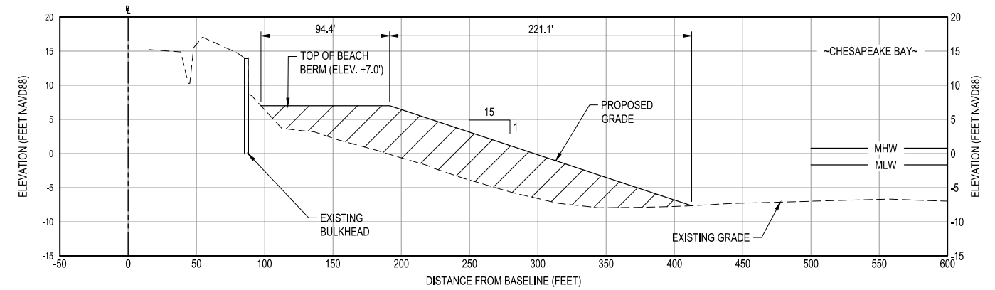
C3 SECTION: STA 15+00 C-302 VERTICAL SCALE: 1"=10' HORIZONTAL SCALE: 1"=50'
