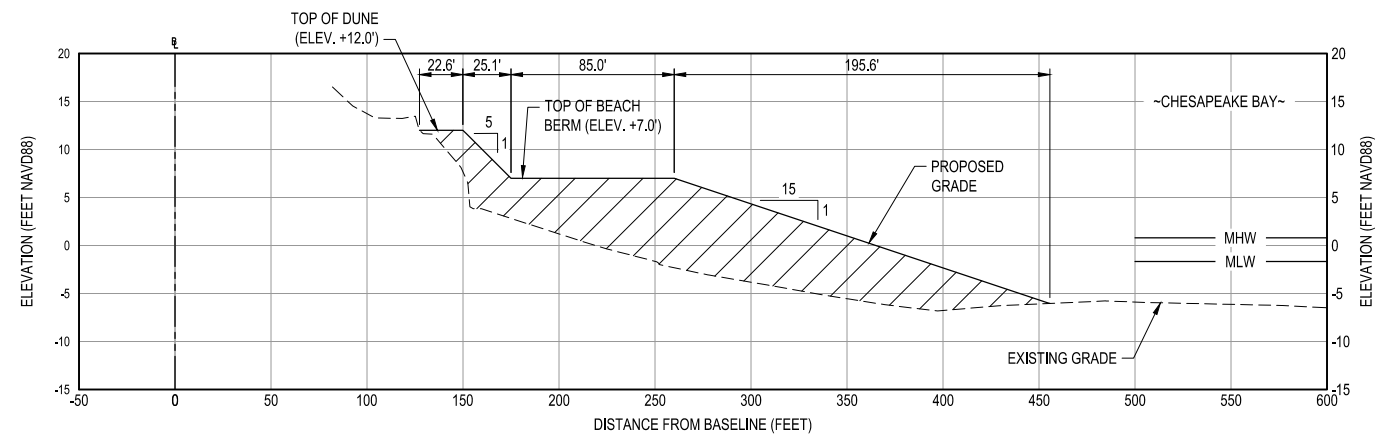
B1 SECTION: STA 25+00 C-302 VERTICAL SCALE: 1"=10' HORIZONTAL SCALE: 1"=50'
