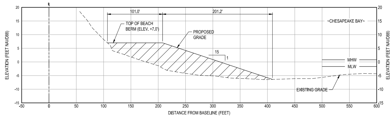
A3 SECTION: STA 35+00 C-301 VERTICAL SCALE: 1"=10' HORIZONTAL SCALE: 1"=50'
