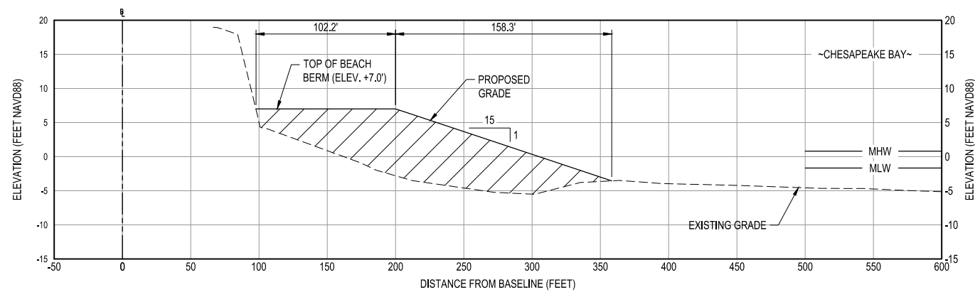
B3 SECTION: STA 40+00 C-301 VERTICAL SCALE: 1"=10' HORIZONTAL SCALE: 1"=50'
