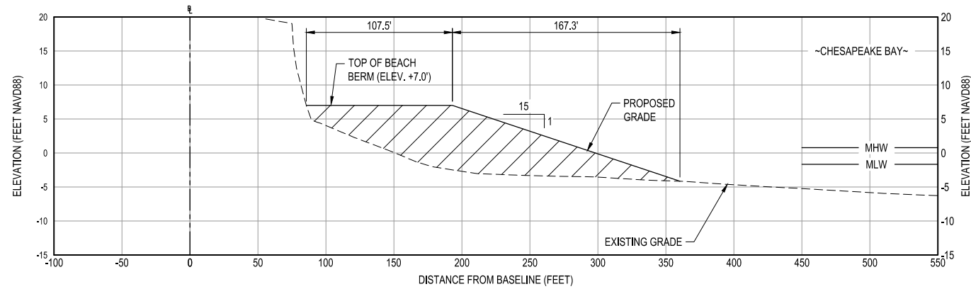
C3 SECTION: STA 45+00 C-301 VERTICAL SCALE: 1"=10' HORIZONTAL SCALE: 1"=50'
