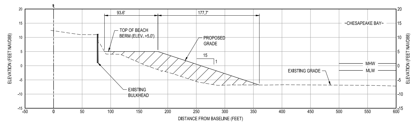
B3 SECTION: STA 10+00 C-302 VERTICAL SCALE: 1"=10' HORIZONTAL SCALE: 1"=50'
