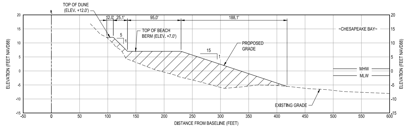
C1 SECTION: STA 30+00 C-302 VERTICAL SCALE: 1"=10' HORIZONTAL SCALE: 1"=50'
