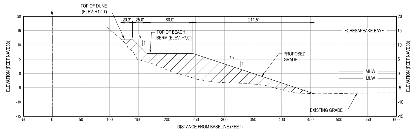
A1 SECTION: STA 20+00 C-302 VERTICAL SCALE: 1"=10' HORIZONTAL SCALE: 1"=50'
